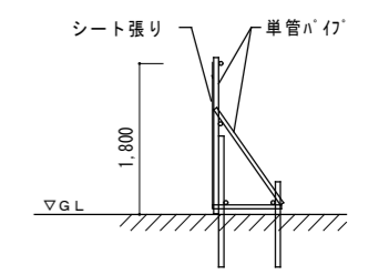
仮囲B断面図(参考) 1/50
