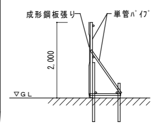
仮囲A断面図(参考) 1/50
